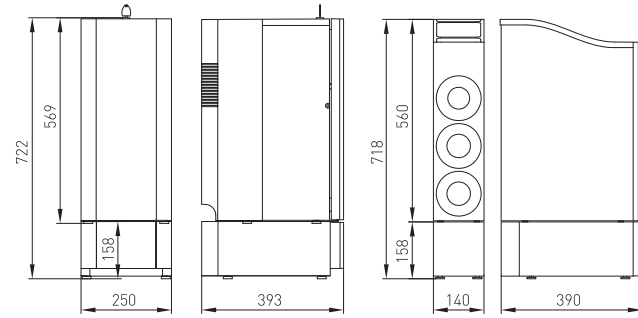
Bijgeplaatste koelunit met onderzetunit
